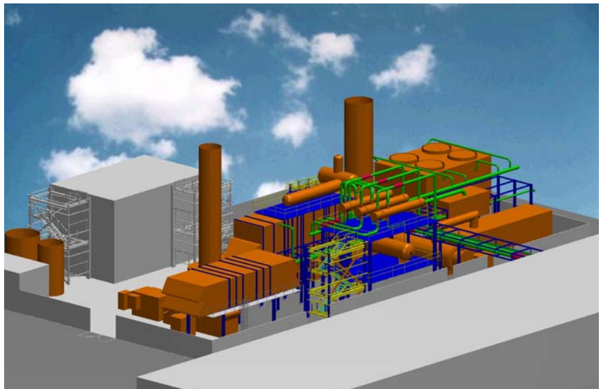
In questo rendering 3D l'aspetto della futura centrale di Cogenerazione Barilla di Pedrignano
